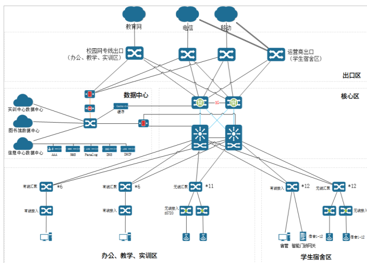
图 3-10 2019 年改造后的校园网络拓扑图
